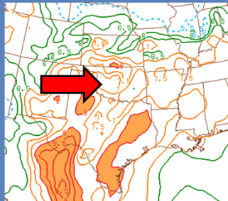
MLLR: 7-7.5°C/km
