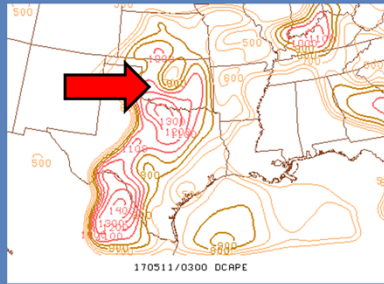
170511/0300 DCAPE DCAPE: 800 j/kg
